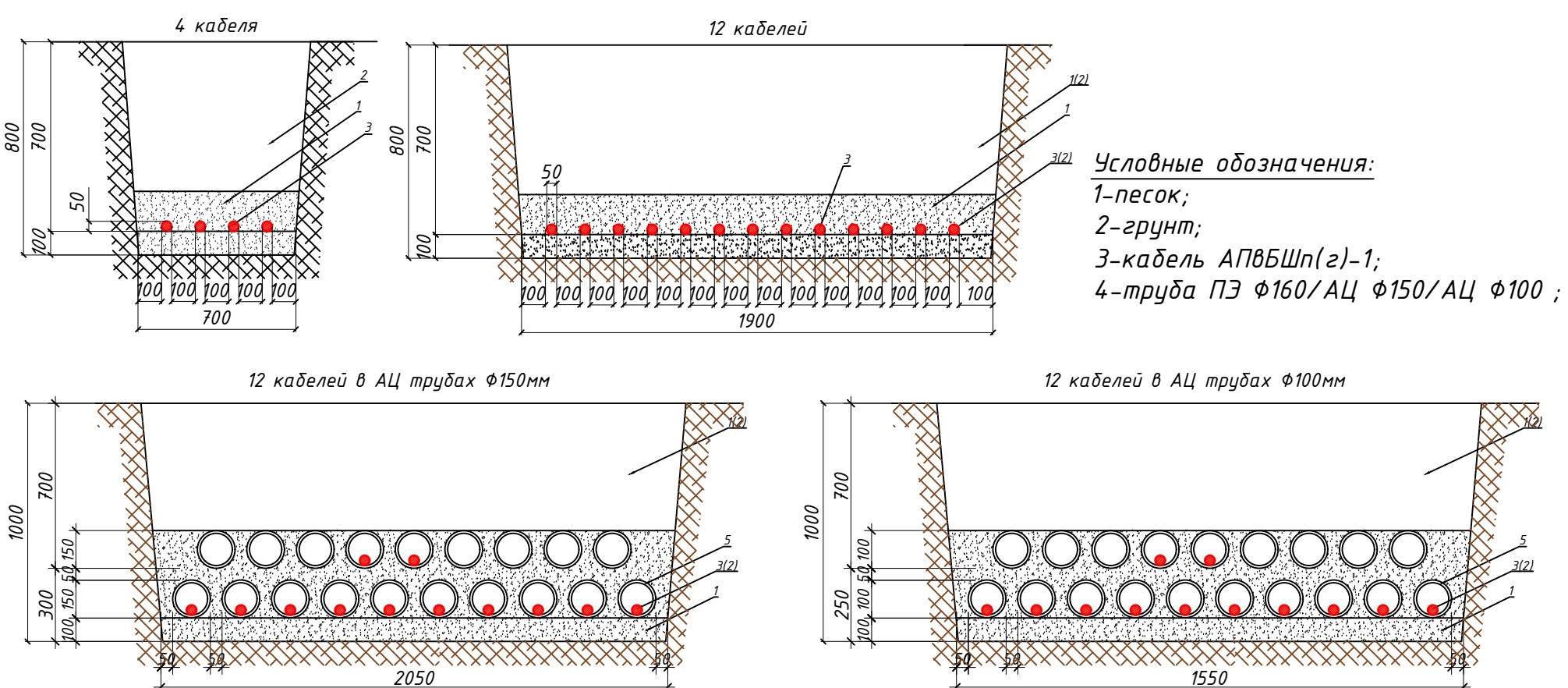
Разрез траншеи
